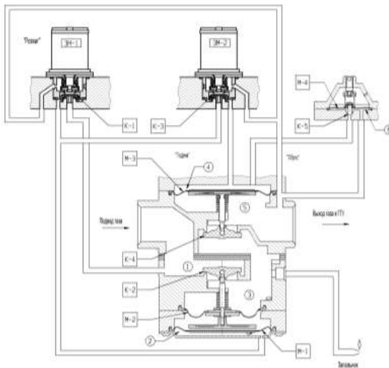
Рисунок 10 – Схема пневматическая газового блока
