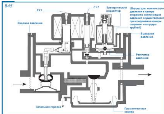
Рисунок 12 – Устройство клапана в разрезе
