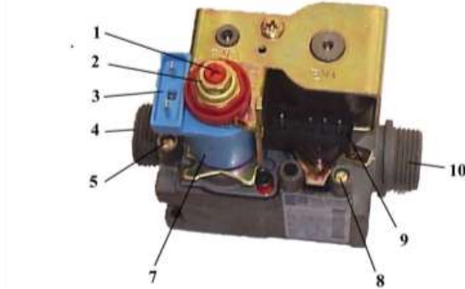
Рисунок 11 – Устройство клапана SIT 845 SIGMA или его аналога
