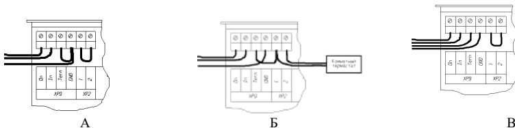
Рисунок 6 – Схема электрическая соединений
