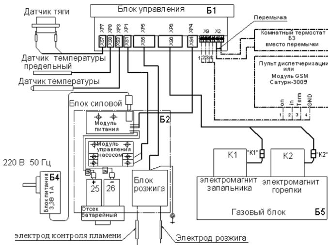
Рисунок 6 – Схема электрическая соединений
