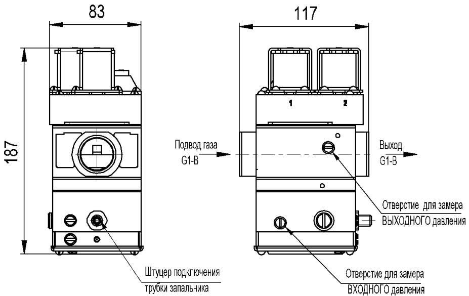
Рисунок 8 – Газовый блок
