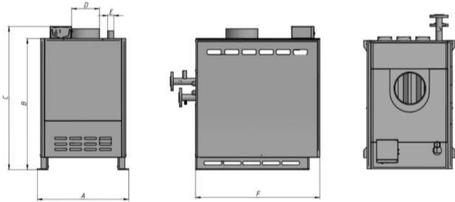
1 – Габаритные размеры
