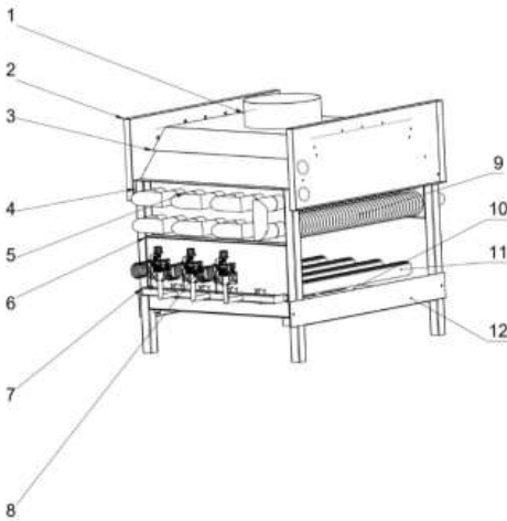
Рисунок 2 – Устройство котла
